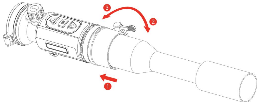
Abbildung 2-7 Tageslichtzielfernrohr montieren
