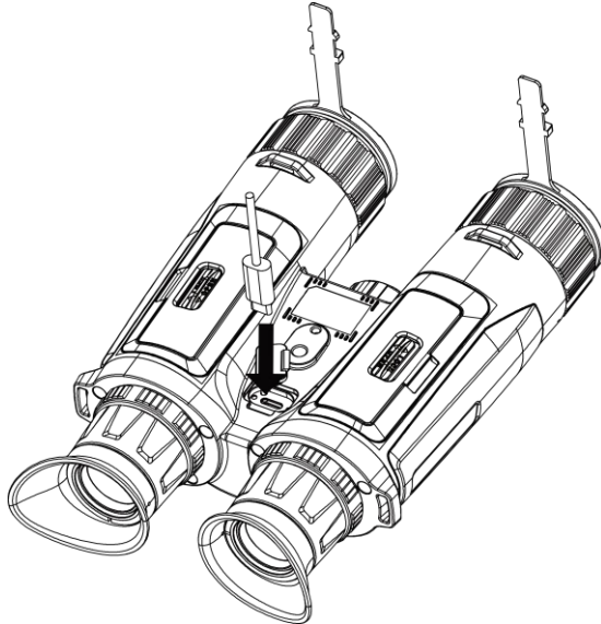
Abbildung 2-4 Kabelanschluss
