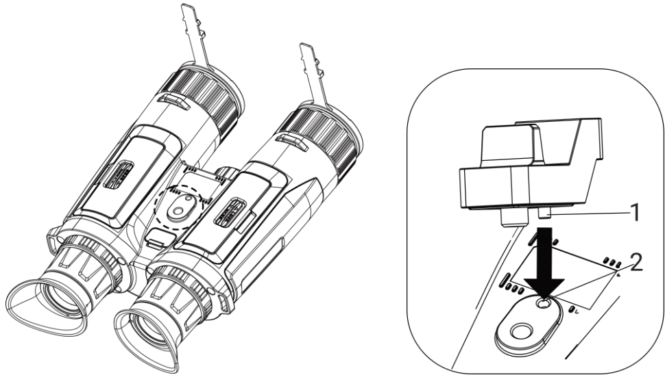
Abbildung 2-8 Adapter suchen und einsetzen
