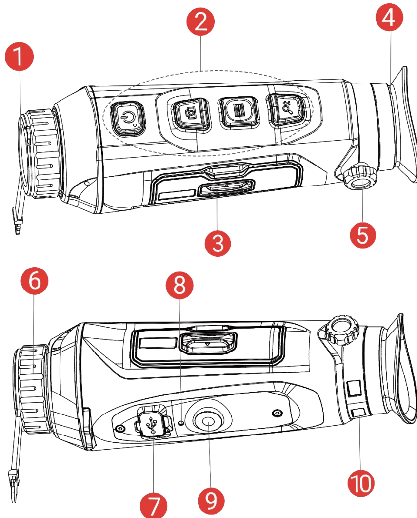
Abbildung 1-1 Aufbau
