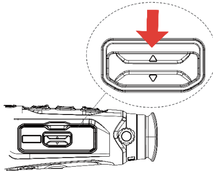
Abbildung 2-1 Die Abdeckung entriegeln
